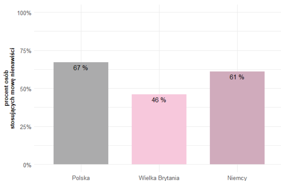
Wykres 4. Procent osób deklarujących stosowanie mowy nienawiści wymierzonej w osoby pobierające zasiłki w Polsce, Wielkiej Brytanii i Niemczech. Na wykresie zagregowano wszystkie odpowiedzi oprócz „1 - nigdy”.
